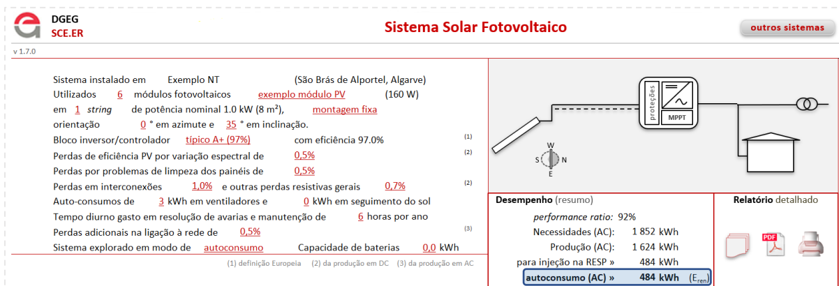
Figura 6 – Output da simulação 1
