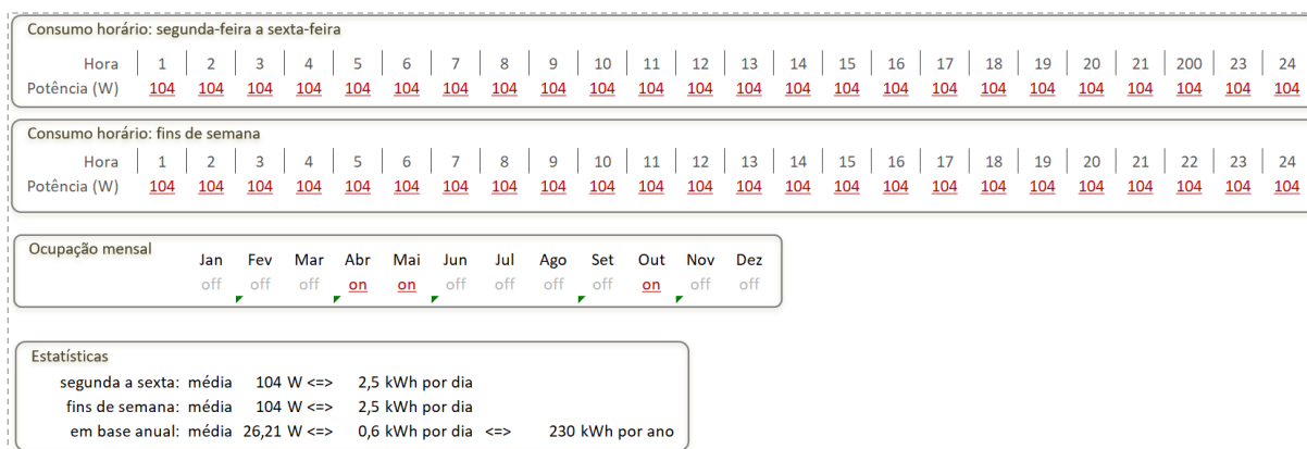
Figura 5 – Perfil de consumo de energia elétrica da simulação 3
